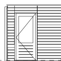
ZIJGEREL 1:100 bwnr get.: 535, 539
