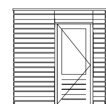
ZIJGEREL 1:100 bwnr get.: 540
