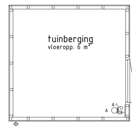
plattegrond 150 bwnr get.: 533
