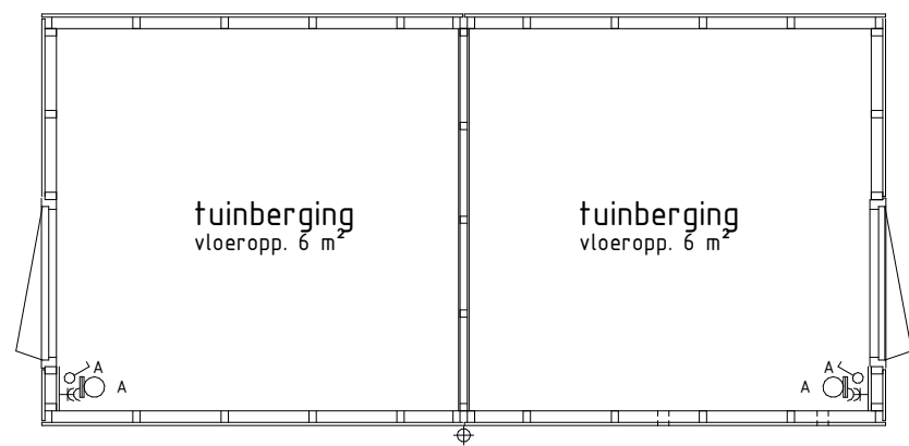
plattegrond 150 bwnr get.: 534, 538 bwnr get.: 535, 539
