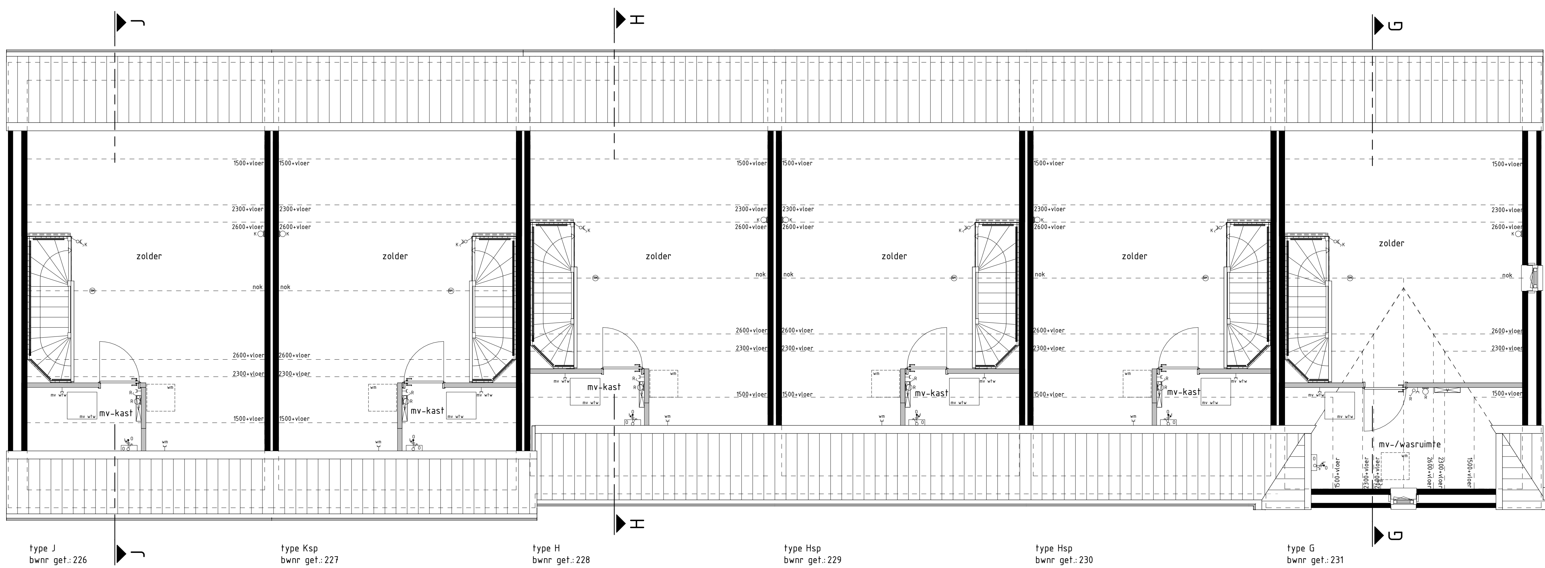
2e VERDIEPING
