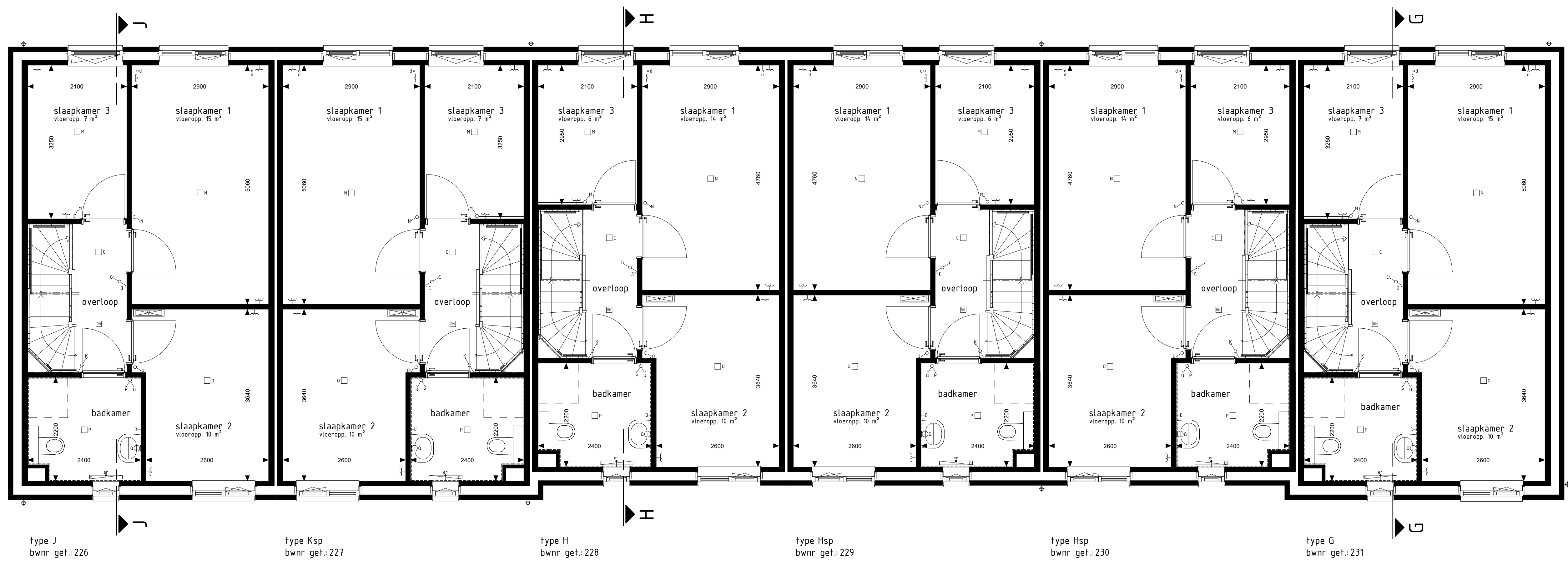
1e VERDIEPING
